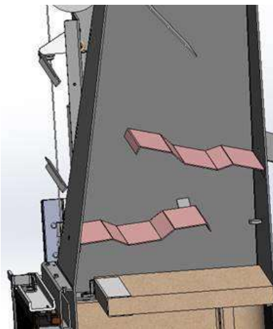
Figura nº27 - Posição atual dos defletores
