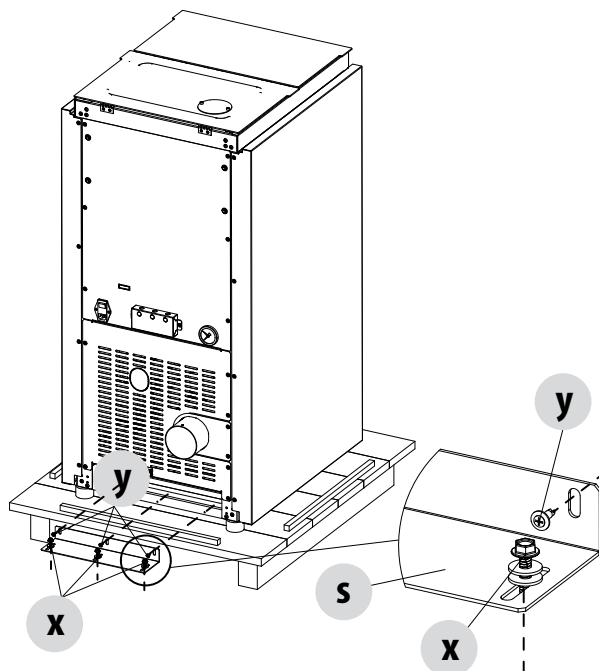
Figura 2 - Remoção da armação traseira
