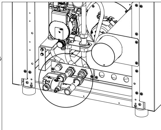
VÁLVULA ANTICONDENSAÇÃO A INSTALAR EM SELECTA 15/20/25HQ
