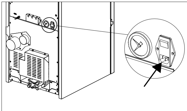
BRANCHEMENT ÉLECTRIQUE
