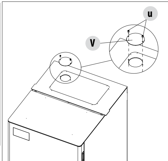
CHARGEMENT AUTOMATIQUE
