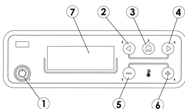
Fig. 7 - Painel de comandos
