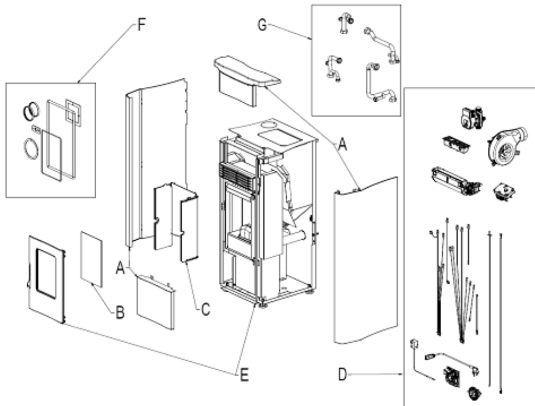
Fig. 1 - Desenho explodido
