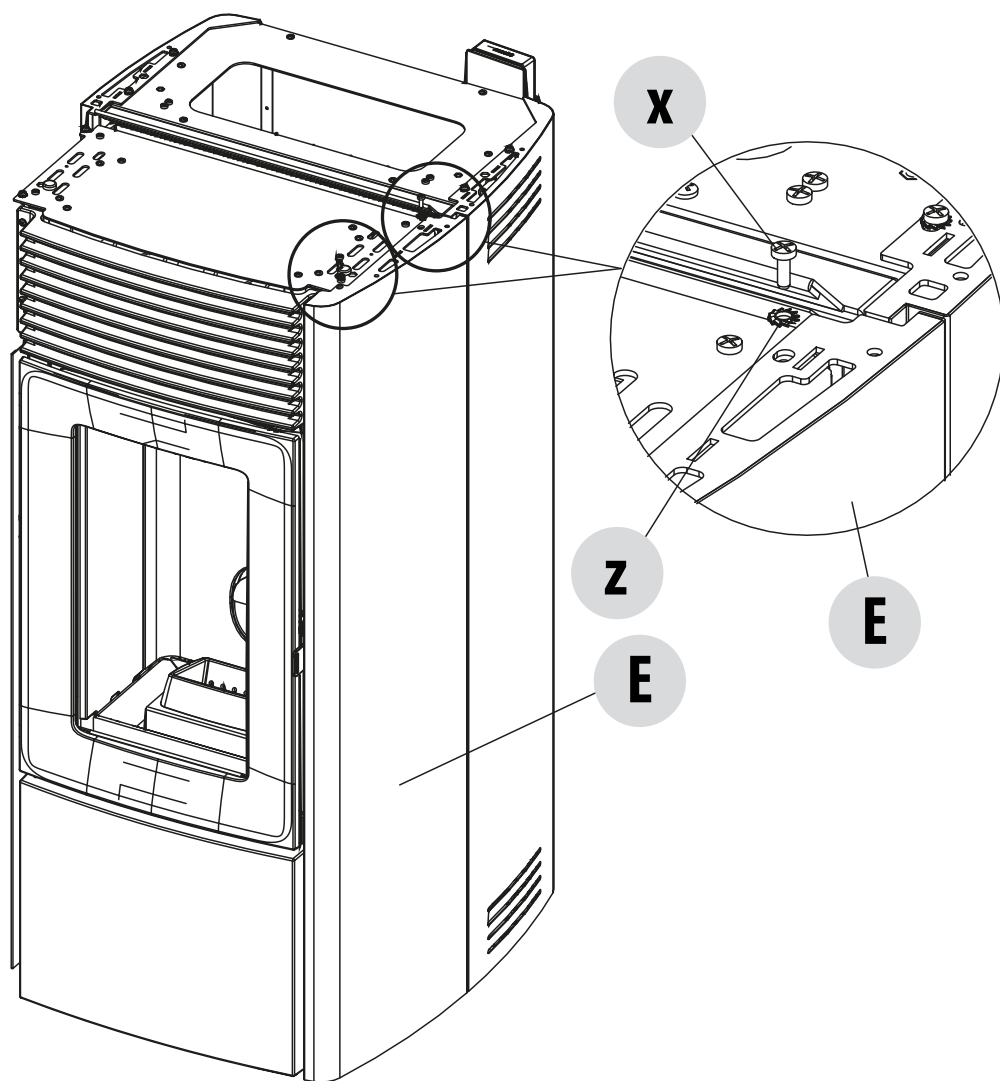
FIXAÇÃO SUPERIOR DO PAINEL EM METAL
