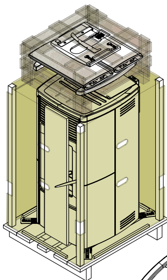
EMBALAGEM STAR COM REVESTIMENTO EM CERÂMICA (EM CIMA)
