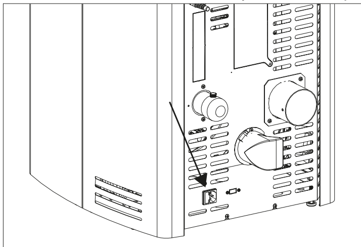
LIGAÇÃO ELÉTRICA DA ESTUFA
