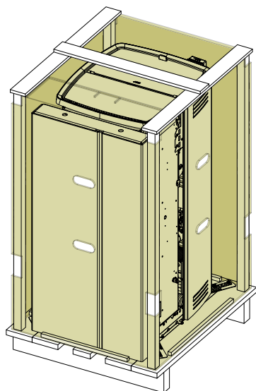
EMBALAGEM EGO COM REVESTIMENTO EM AÇO
