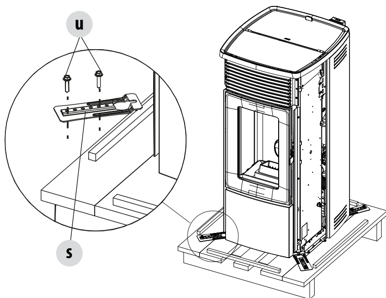
REMOÇÃO DOS ELEMENTOS DE FIXAÇÃO (NA FIGURA: ESTUFA EGO)
