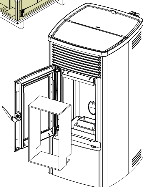
REMOÇÃO DA EMBALAGEM DA FORNALHA
