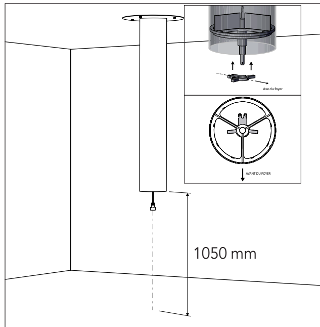
PT Fixar o limitador de rotação no eixo da tubagem, como indicado acima, respeitando a altura indicada no passo seguinte.
