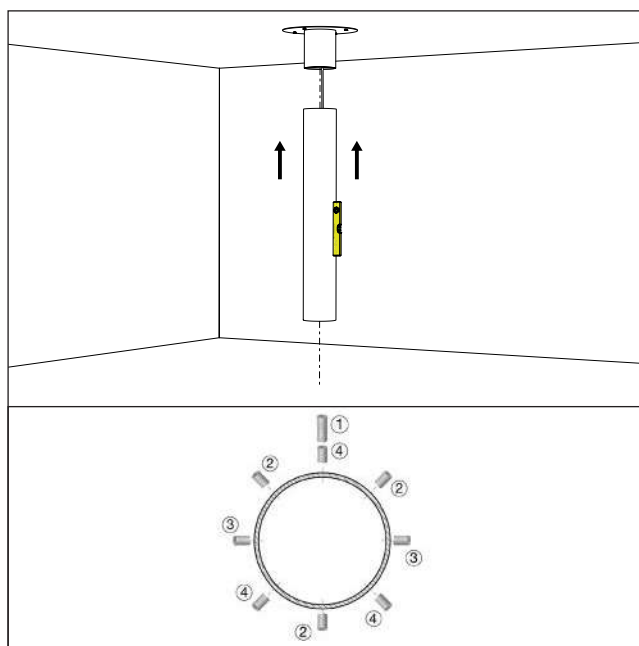
PT Fixar a(s) conduta(s) respeitando a ordem de aperto mostrada.
