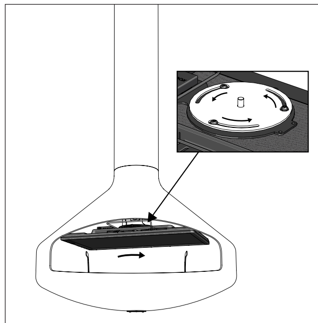
PT Instalar a placa inserindo os parafusos nos locais específicos.
