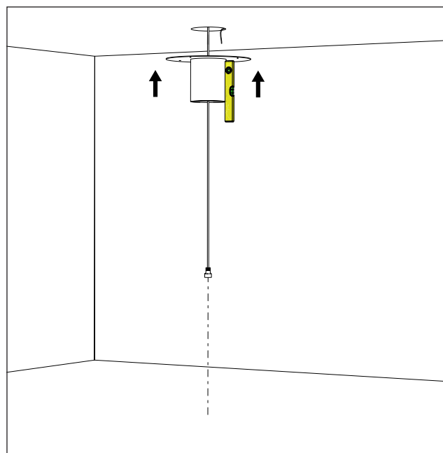
PT Fixar a platina com nível.
