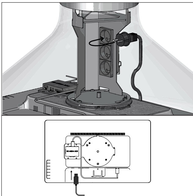
PT Ligar o cabo de alimentação da placa.
