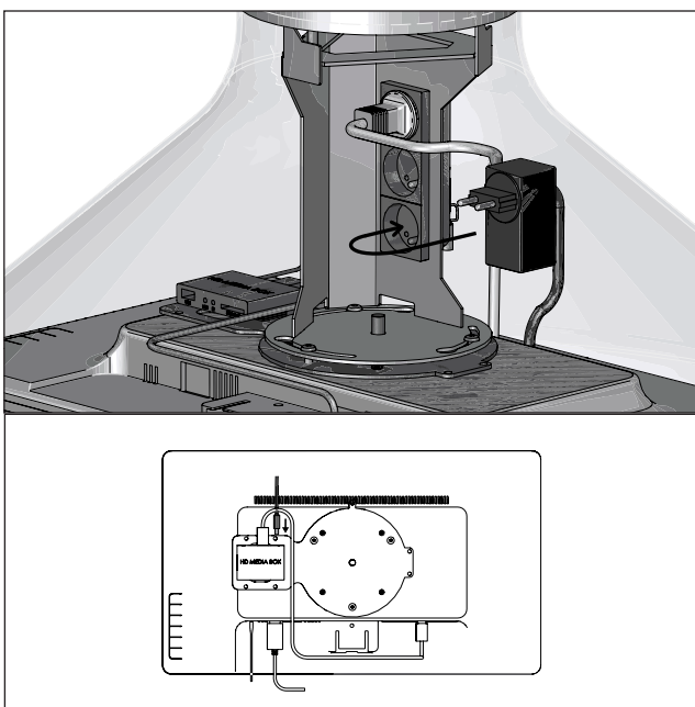
PT Ligar o cabo de alimentação ao reproduztor.
