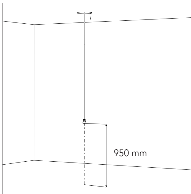
PT Instale um cabo de alimentação com uma ligação à terra fêmea na extremidade.
