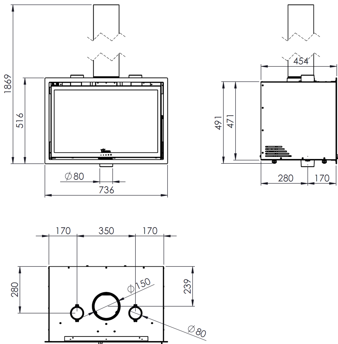
Figura nº1 - Dimensões em mm do aparelho NIVE 700 STAR
