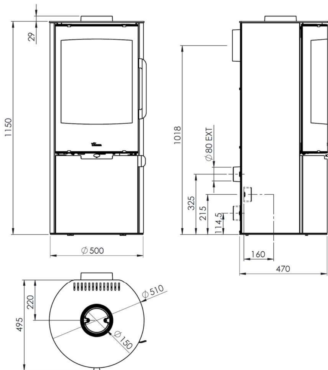
Figura nº1 - Dimensões em mm de MAYA e MAYA Visión
