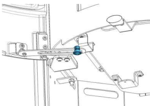
Figura nº22 - Passo 2. Desmontar eixo
