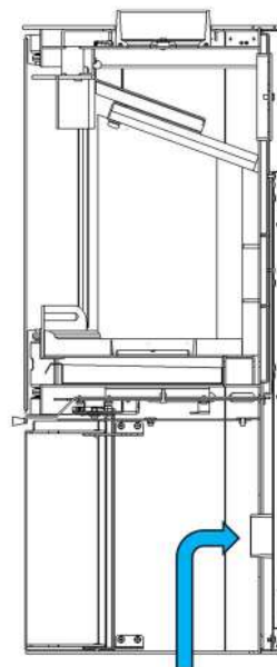
Figura nº10 - OPÇÃO 3 Condução de ar para a câmara de combustão
