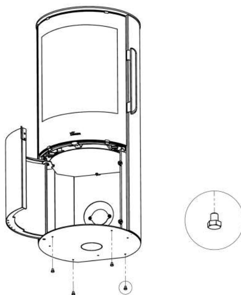
Figura nº20 - Instalação dos pés de nivelamento
