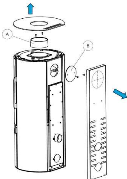
Figura nº5 - Trocar os componentes (A) e (B) para saída de fumos posterior
