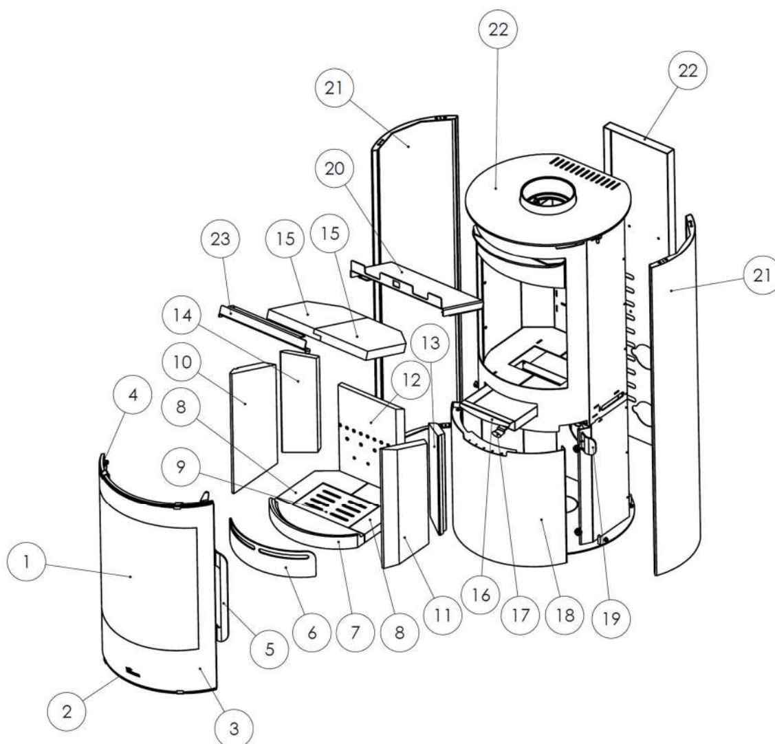
Figura nº2 - Explosão de peças MAYA Visión
