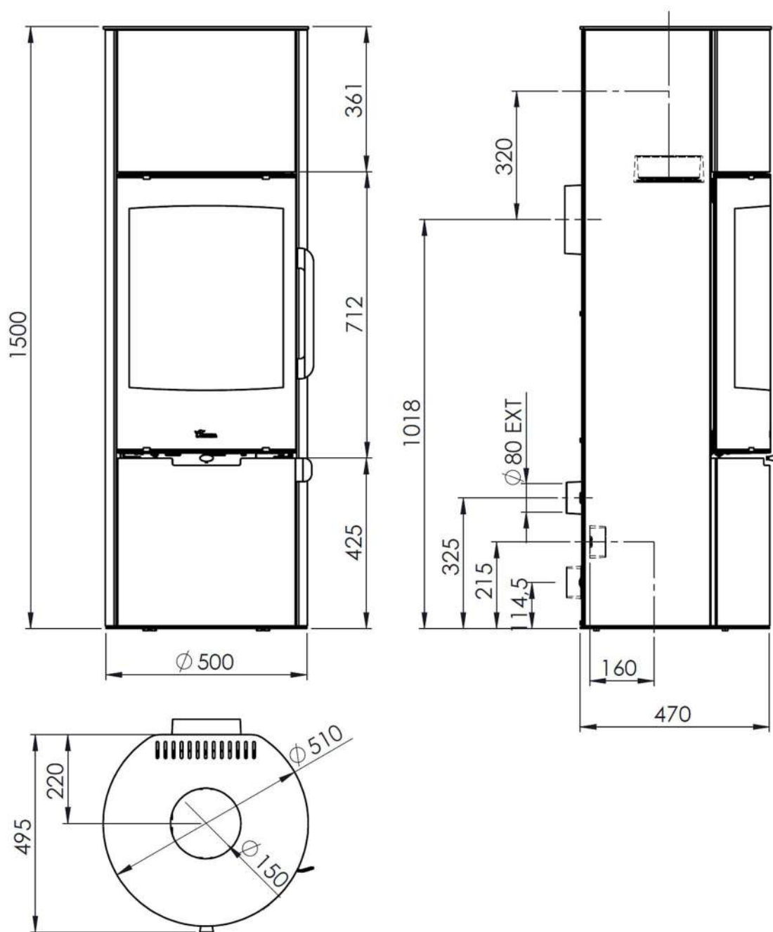
Figura nº2 - Dimensões em mm de MAYA ACU e MAYA ACU Visión
