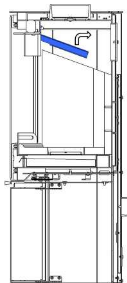
Figura nº19 - Desmontar defletor de aço
