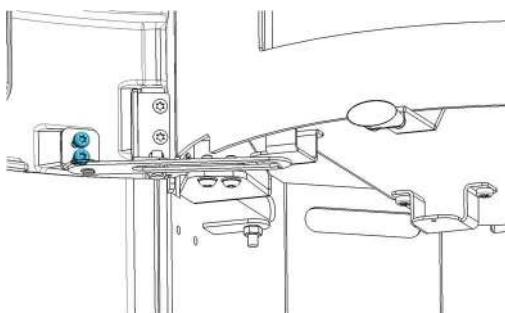
Figura nº23 - Passo 3. Desmontar parafusos do suporte da porta
