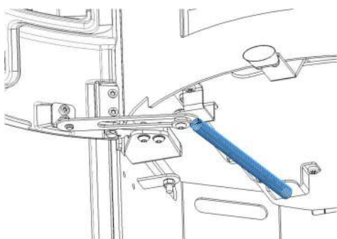
Figura nº21 - Passo 1. Desmontar mola
