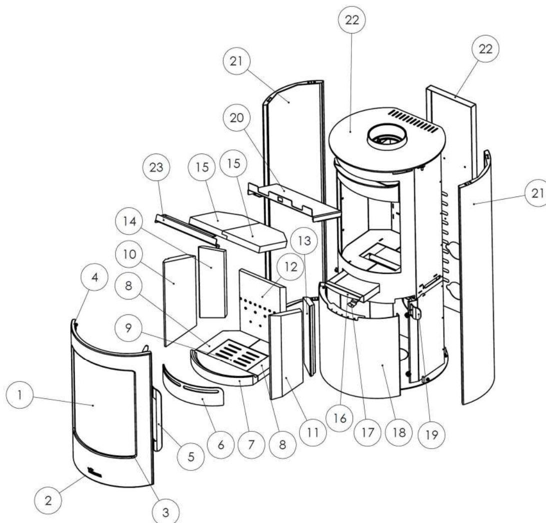
Figura nº1 - Explosão de peças MAYA
