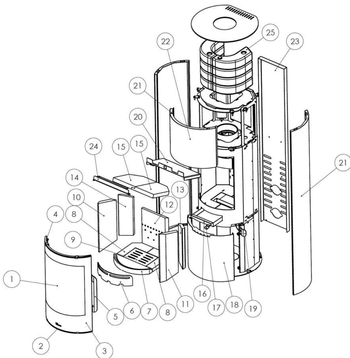
Figura nº4 - Explosão de peças MAYA ACU Visión
