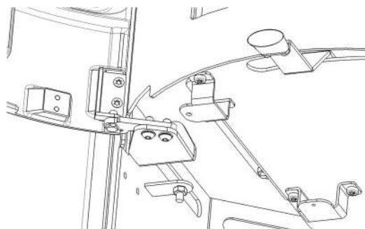
Figura nº24 - Passo 4. Retirar mecanismo
