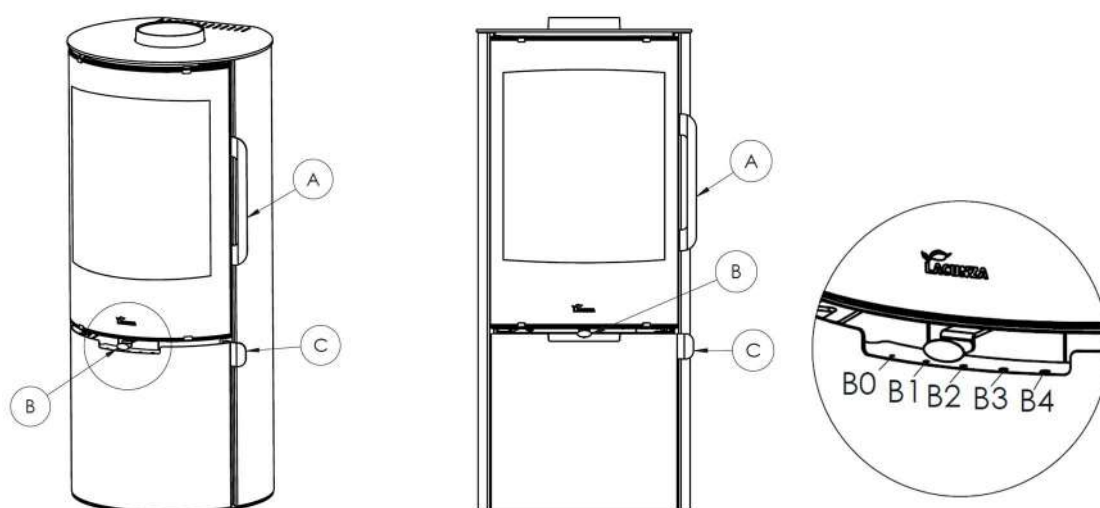
Figura n°15 - Elementos de funcionamento do aparelho
