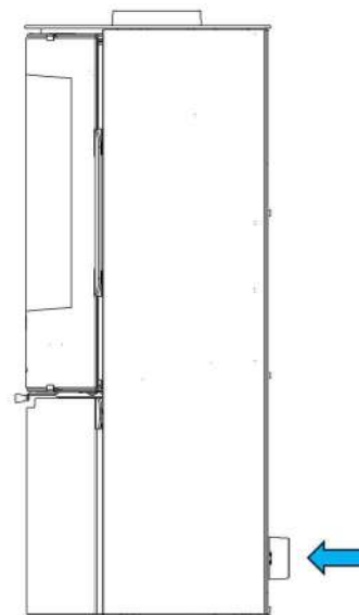
Figura nº8 - OPÇÃO 2 Condução de ar para a câmara de combustão
