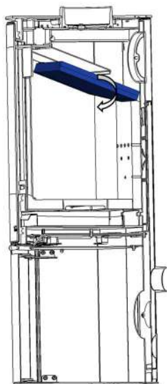
Figura nº18 - Retirar vermiculite
