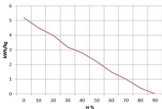
Figura n°14 - Relação entre humidade e poder calorífico da lenha.
