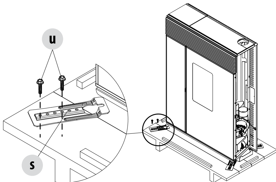
RIMOZIONE STAFFE DI FISSAGGIO
